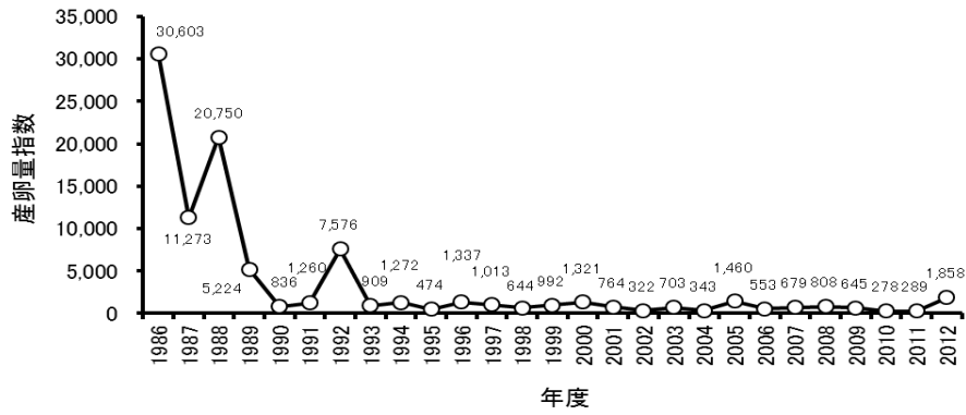
図6-4 根室海峡におけるスケトウダラ産卵量指数の経年変化 図出典:平成24年度道総研釧路水産試験場事業報告書
