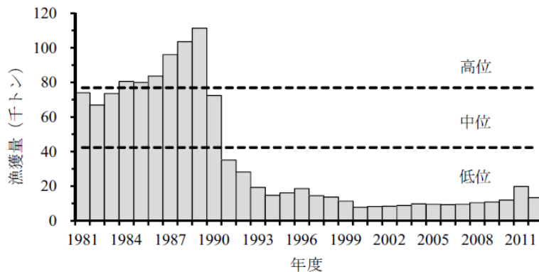
図6-3 スケトウダラ根室海峡の資源水準値
